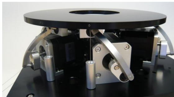
パラレルリンク構造の位置決めステージ
